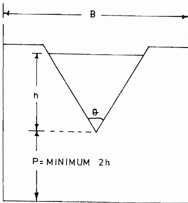
FIG. 25.1 : V - NOTCH
