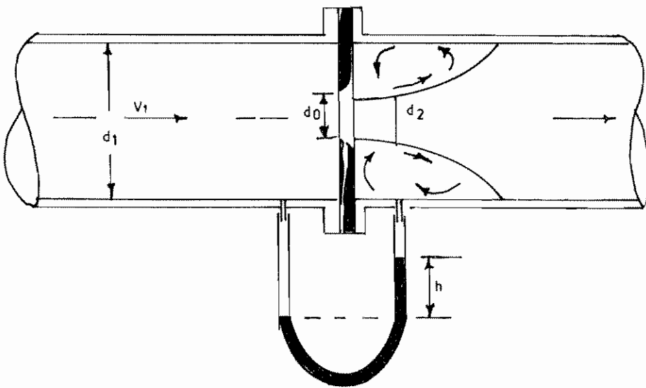
FIG. 25.12 :ORIFICE METER
